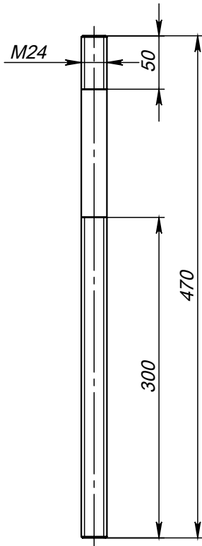
Поз.5 (Шпилька)
